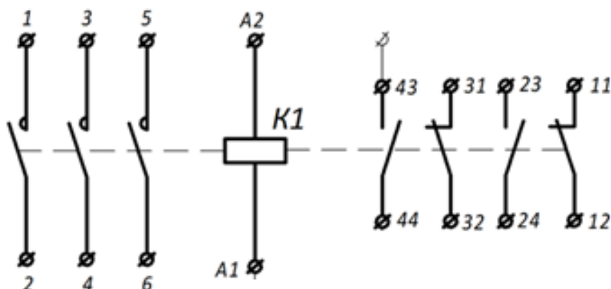
Рисунок 1. Схема пускателя без теплового реле
